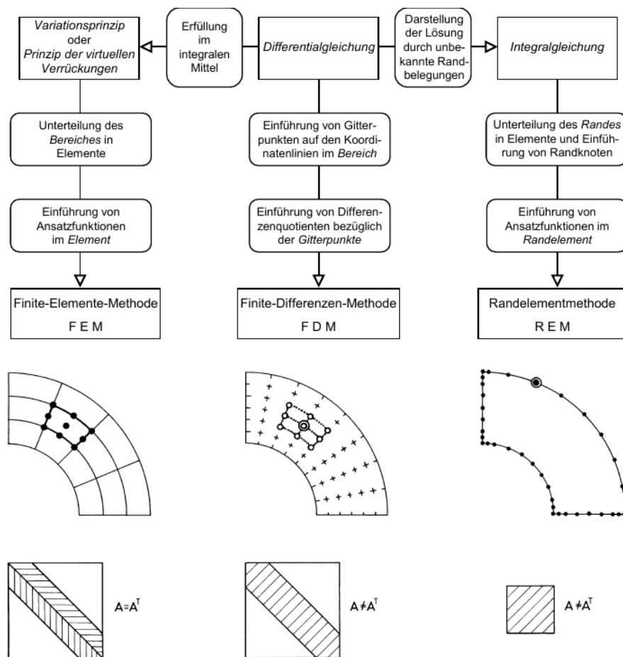
Figure 1.6: Vergleich verschiedener Diskretisierungsverfahren nach Knothe and Wessels [1991]
