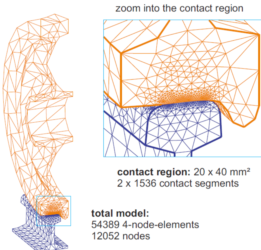
Figure 1.31: Geometrieapproximation am Beispiel der Diskretisierung eines Eisenbahnrades Nackenhorst [2022].
