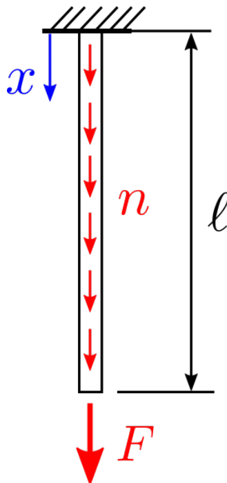
Figure 1.18: Stab unter Eigengewicht und externer Kraft.
