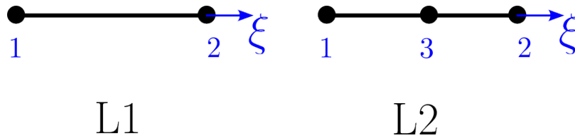
Figure 1.42: 1D-Elemente mit linearer und quadratischer Ansatzfunktion
