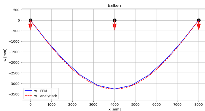
Figure 1.26: Gegenüberstellung der analytischen Verschiebungslösung mit der FEM-Lösung.
