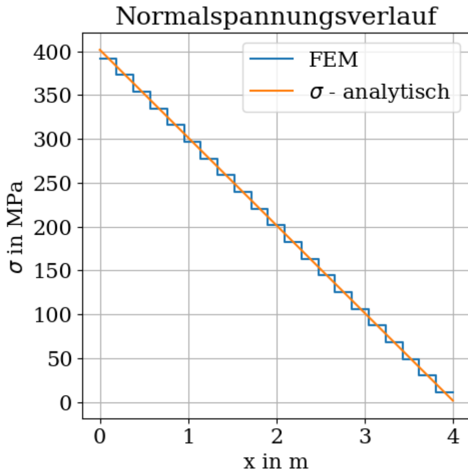
Figure 1.20: Ergebnisse für die Normalspannung in einem Stab unter Eigengewicht mit einer erhöhten Netzfeinheit.
