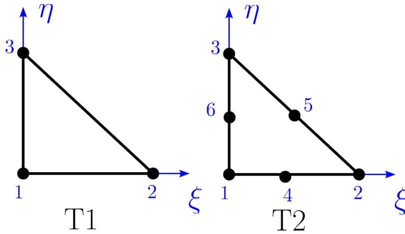
Figure 1.47: Dreieck-Elemente mit linearen (T1) und quadratischen (T2) Formfunktionen.
