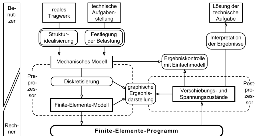
Figure 1.1: Einordnung numerischer Simulation in den Konstruktionsprozess nach Knothe and Wessels [1991]
