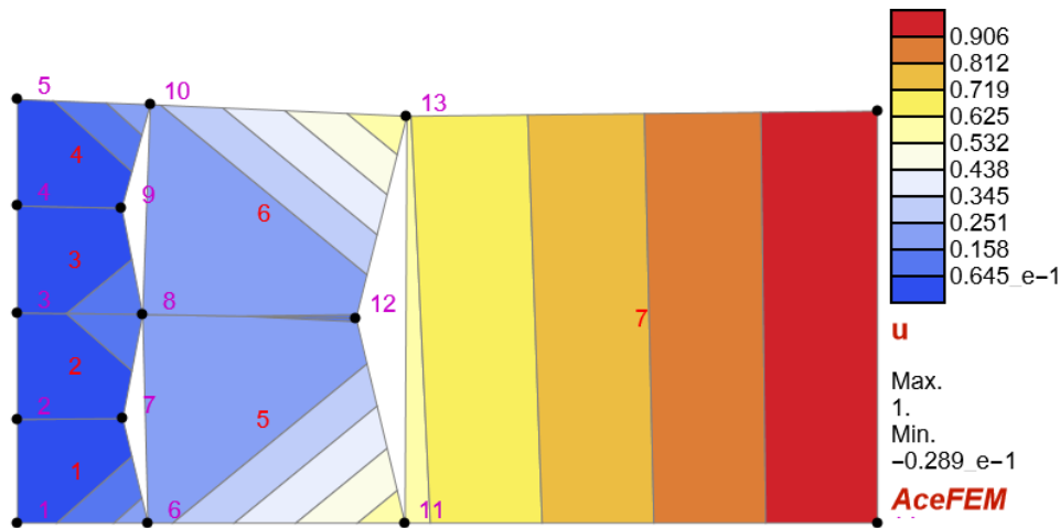
Figure 1.34: Verschiebungsfeld bei einer nicht-konformen Netzstruktur.
