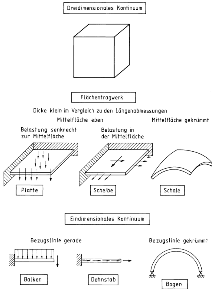
Figure 1.14: Übersicht über die Klassifizierung von Strukturvereinfachungen nach Knothe and Wessels [1991]
