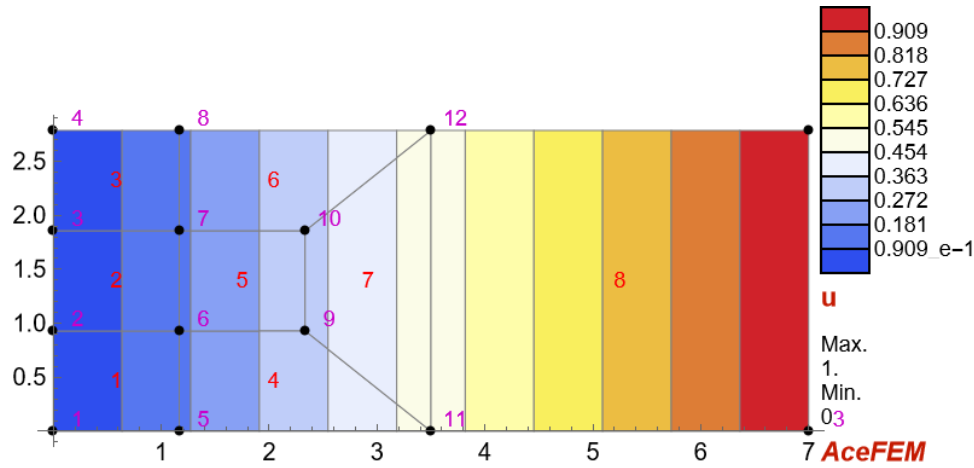
Figure 1.38: Übergangselementschicht zur lokalen Verfeinerung - Verschiebungsfeld.
