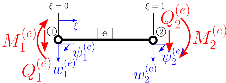
Figure 1.23: Balkenelement mit lokalen Freiheitsgraden
