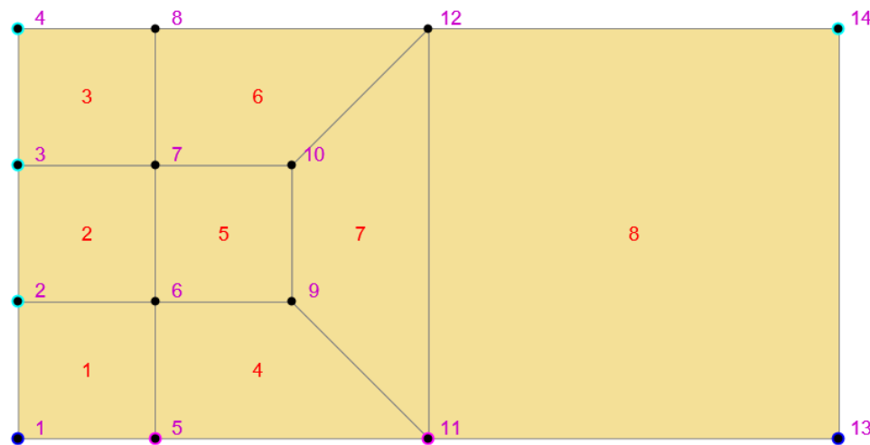
Figure 1.37: Übergangselementschicht zur lokalen Verfeinerung.
