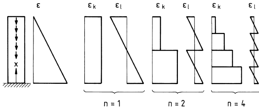
Figure 1.39: Mit steigender Elementanzahl wird der konstante Term der Schnittkraft dominant (Knothe and Wessels [1991]).
