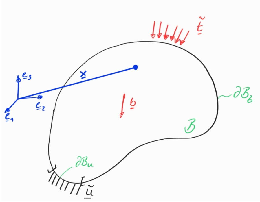
Figure 1.17: Körper \mathcal{B} unter Einwirkung der externen Oberflächenkraft \tilde{\mathbf{t}} und der Volumenlast \mathbf{b}
