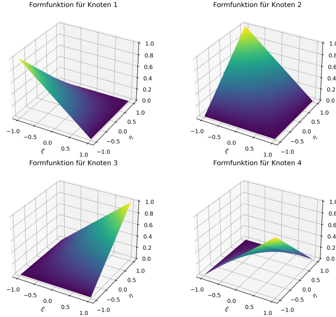
Figure 1.44: Bilineare Formfunktionen für 2D-Rechteck-Elemente.
