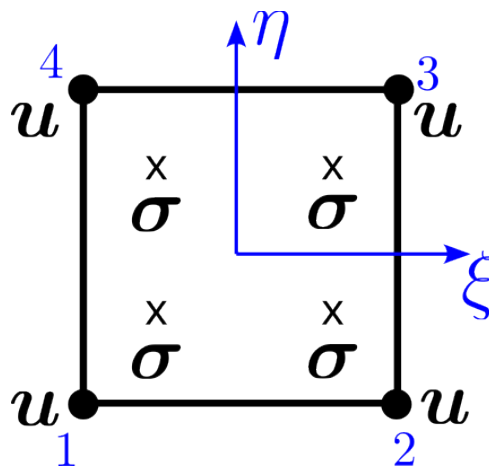
Figure 1.55: Unterschied zwischen primären und sekundären Größen im Postprocessing.
