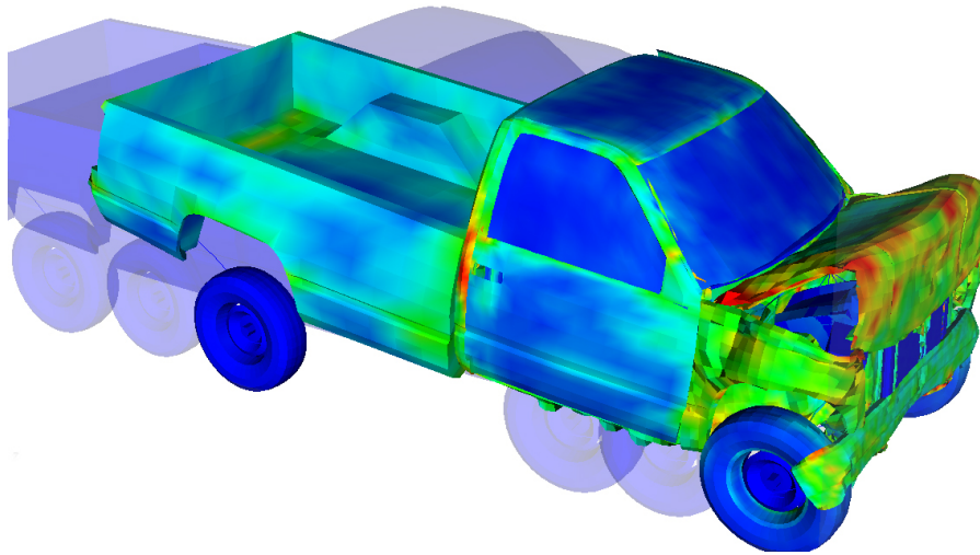
Figure 1.11: FEM Crash-Simulation eines Pickup-Trucks gegen eine starre Wand Quelle
