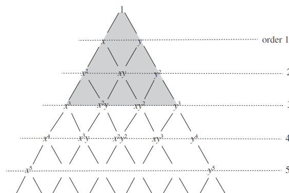
Figure 1.40: Pascal'sches Dreieck für Dreieckselemente (Zienkiewicz et al. [2005])
