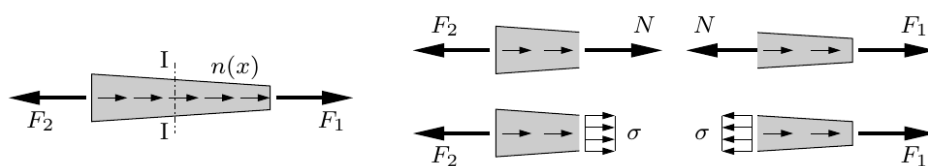
Figure 1.15: Kräftegleichgewicht und Spannungen am geraden Stab nach Wriggers et al. [2006]
