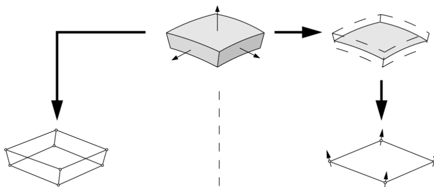
Figure 1.12: FEM-Diskretisierung von Schalenelementen als degenerierte Volumenelemente (links) oder über eine Mittelflächendarstellung (rechts). Wriggers [2008]
