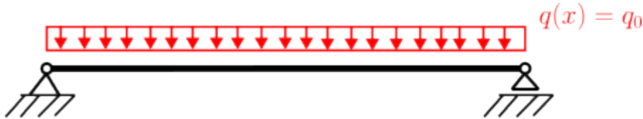
Figure 1.24: Statisch bestimmt gelagerter Balken mit konstanter Streckenlast
