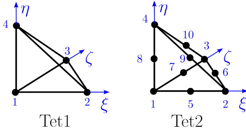
Figure 1.50: Tetraedrische Elemente mit linearen (Tet1) und quadratischen (Tet2) Formfunktionen.
