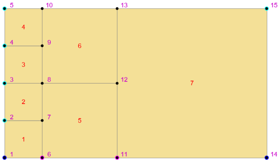
Figure 1.33: Verletzung der Stetigkeitsanforderung in der Finite-Elemente-Methode.
