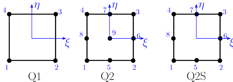
Figure 1.43: 2D-Rechteck-Elemente mit linearer und quadratischer Ansatzfunktion
