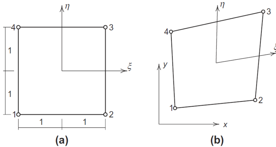
Figure 1.32: Abbildung des Elternelementes auf die reale Geometrie (Zienkiewicz et al. [2005]).
