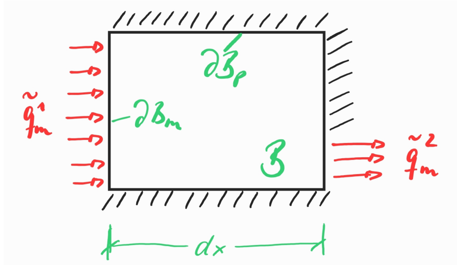
Figure 1.7: Ein- und Ausfluss eines infinitesimalen Volumenelementes Austausch
