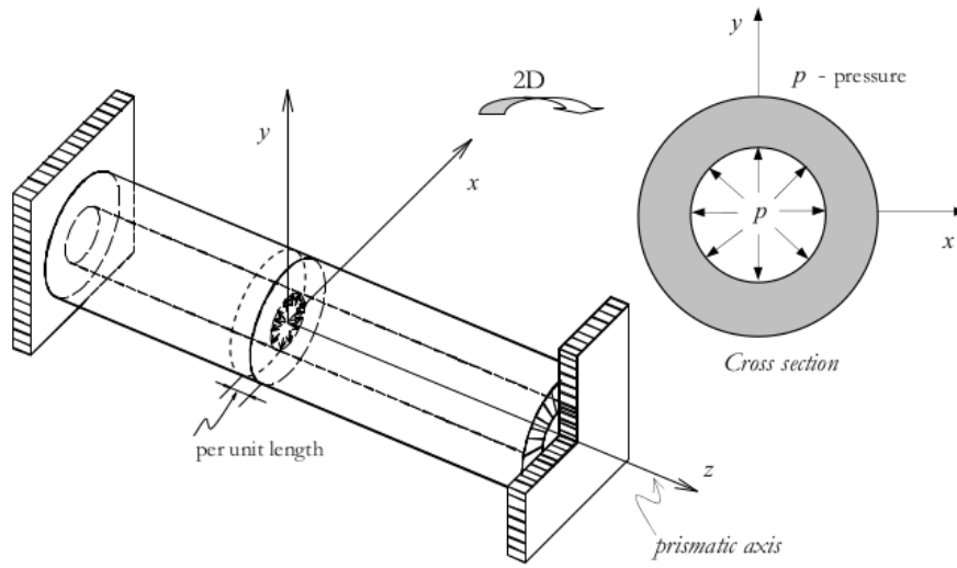
Figure 1.10: Beispiel für das Auftreten eines ebenen Verzerrungszustands Chaves [2013]
