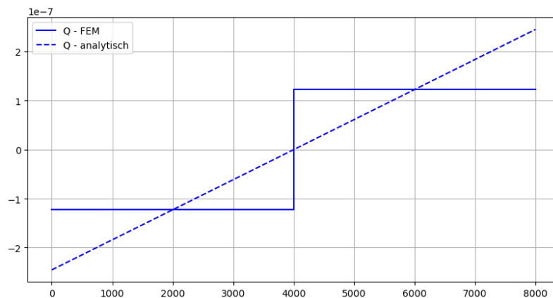
Figure 1.28: Gegenüberstellung der analytischen Lösung für den Querkraftverlauf mit der FEM-Lösung.
