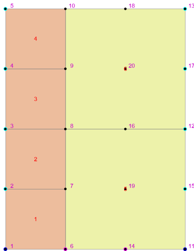
Figure 1.35: Verletzung der Stetigkeitsanforderung in der Finite-Elemente-Methode durch Verwendung von Elementen mit unterschiedlicher Ordnung.
