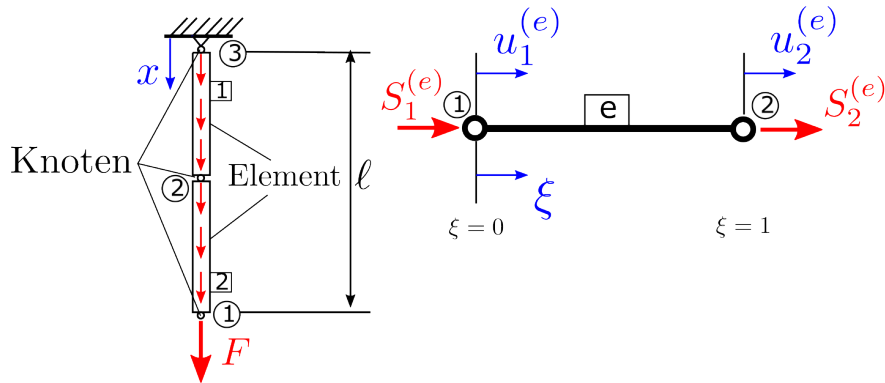
Figure 1.19: Stab unter Eigengewicht und externer Kraft mit Stabelementen diskretisiert.
