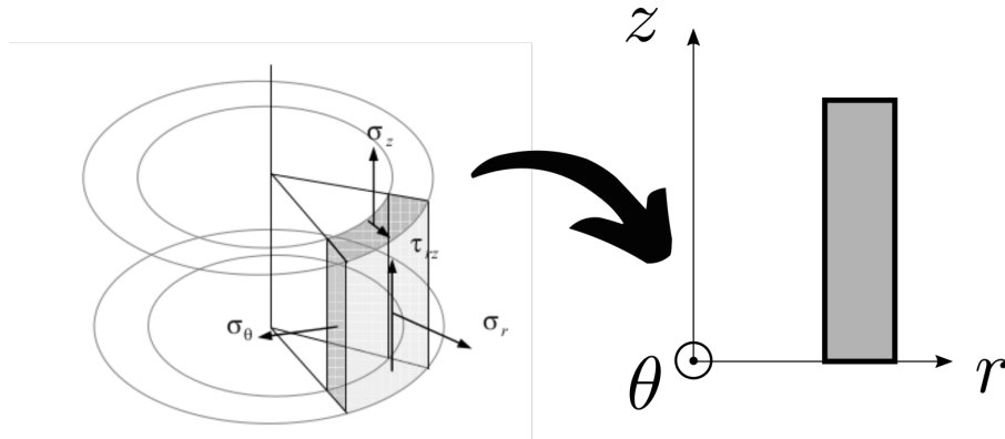
Figure 1.13: Rotationssymmetrischer Körper im Zylinderkoordinatensystem \{r, z, \theta\} . Nach Chaves [2013]
