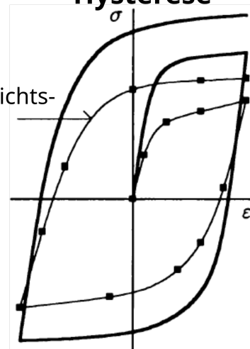
Figure 1.9: Klassifizierung von Materialmodellen anhand ihrer Systemantwort. Abbildung nach Haupt [2013]
