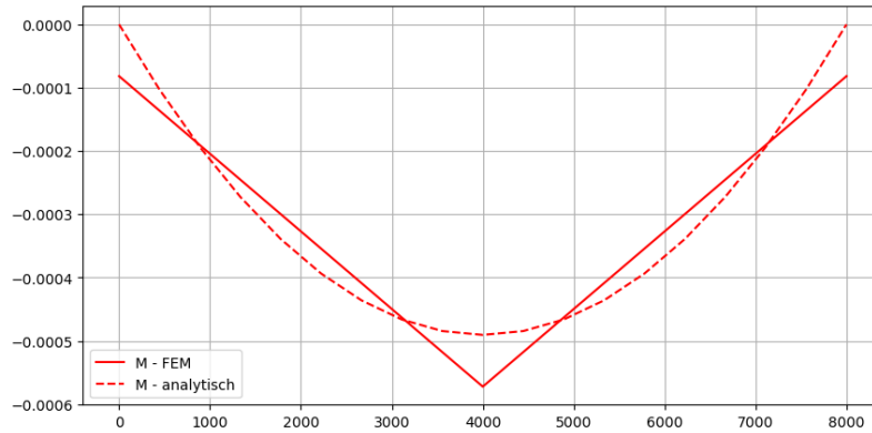
Figure 1.27: Gegenüberstellung der analytischen Lösung des Momentenverlaufs mit der FEM-Lösung.
