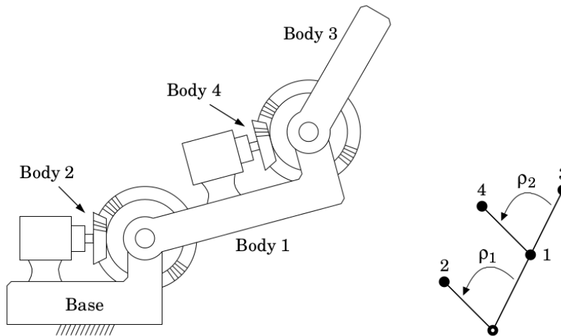
Figure 1.5: Mehrkörperproblem eines zweiarmigen Roboters nach Featherstone [2014]
