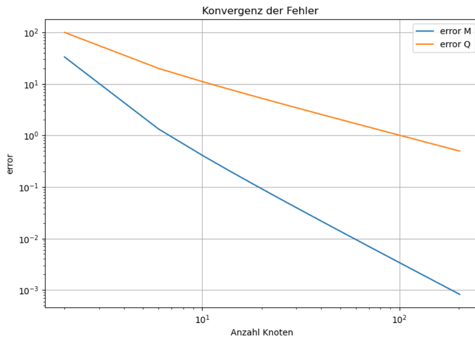
Figure 1.30: Konvergenzverhalten der FEM-Lösung für das Schnittmoment und die Querkraft im doppelt logarithmischen Diagramm.
