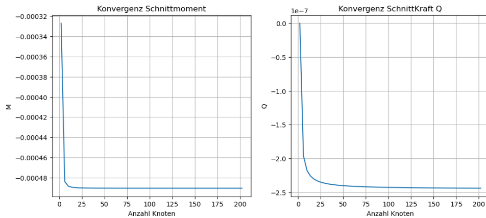
Figure 1.29: Konvergenzverhalten der FEM-Lösung für das Schnittmoment und die Querkraft.
