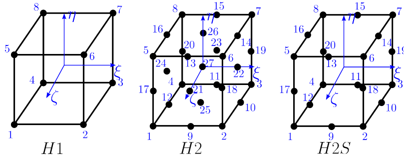
Figure 1.49: 3D-Hexaeder-Elemente mit linearer (8 Knoten) und quadratischer (27 Knoten) Approximation. Zusätzlich ist das 20-Knoten-Hexaeder-Serendipity-Element gezeigt.
