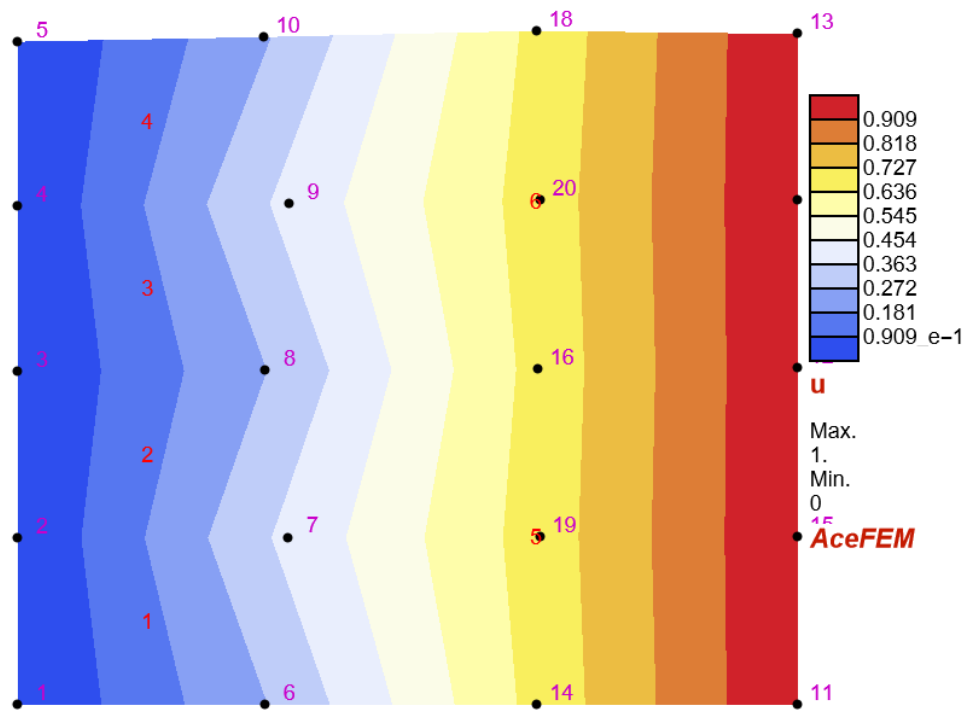
Figure 1.36: Verletzung der Stetigkeitsanforderung in der Finite-Elemente-Methode durch Verwendung von Elementen mit unterschiedlicher Ordnung - Resultierendes Verschiebungsfeld.
