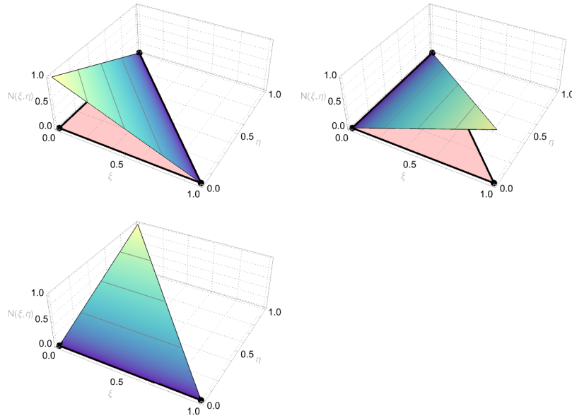
Figure 1.48: Formfunktionen für das Dreieck-Element T1.
